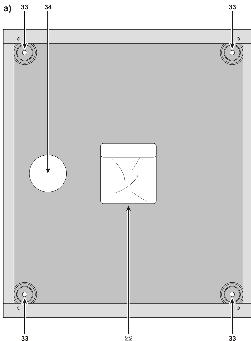
Figura 4 Configuración Máxima del Repetidor J400-REP: a) parte trasera; b) parte frontal (vista interior)
