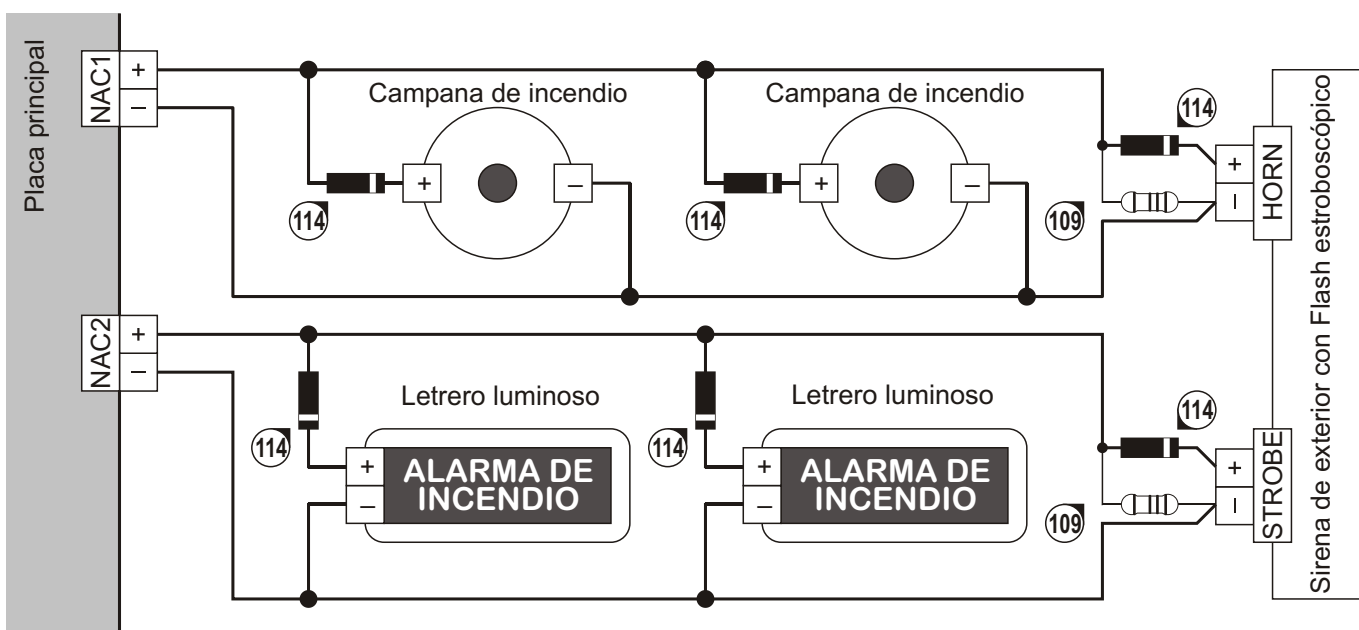
Figura 18 Conexión de dispositivos de Señalización: 109 ) Resistencia Fin de Línea de 3900 ohm, 1/4 W (naranja-blanco-rojo-oro); 114 ) 1N4007 Diodo o similar
