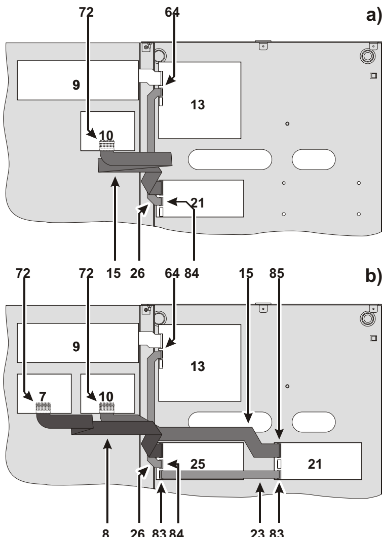
Figura 11 Conexión de UN Módulo Expansor (a) Conexión de DOS Módulos Expansores (b): 7) Tarjeta de Control del Módulo Expansor n°. 2; 8) y 15) Cable plano para conectar la Tarjeta de Control y el Módulo Expansor; 9) Tarjeta de Control Principal; 10) Tarjeta de Control del Módulo Expansor n°. 1; 13) Tarjeta principal; 21) Módulo Expansor n°. 1; 23) y 26) Cable plano para conectar al Módulo Expansor; 25) Módulo Expansor n°. 2; 64) Conector para el Expansor; 72) Terminal para conectar la tarjeta de Control y su respectivo Módulo Expansor (en la cara de los componentes); 83) Terminal para conectar el Módulo Expansor n°. 1 y el Módulo Expansor n°. 2; 84) Terminal para conectar el Módulo Expansor y la Placa Principal; 85) Terminal para conectar la Tarjeta de Control.
