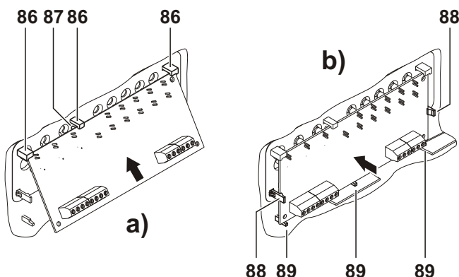
Figura 7 J408: Instalación del Módulo de Extinción
