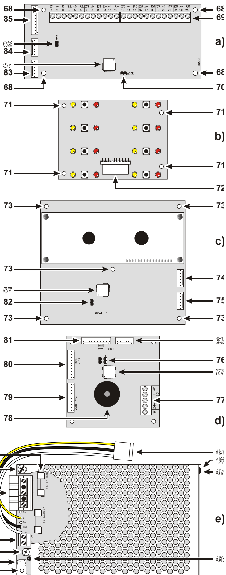
Figura 6 Identificación de las Partes: a) Módulo Expansor; b) Tarjeta de Control del Expansor; c) Módulo Display; d) Interface del Repetidor RS485; e) Fuente de Alimentación de la Central J424
