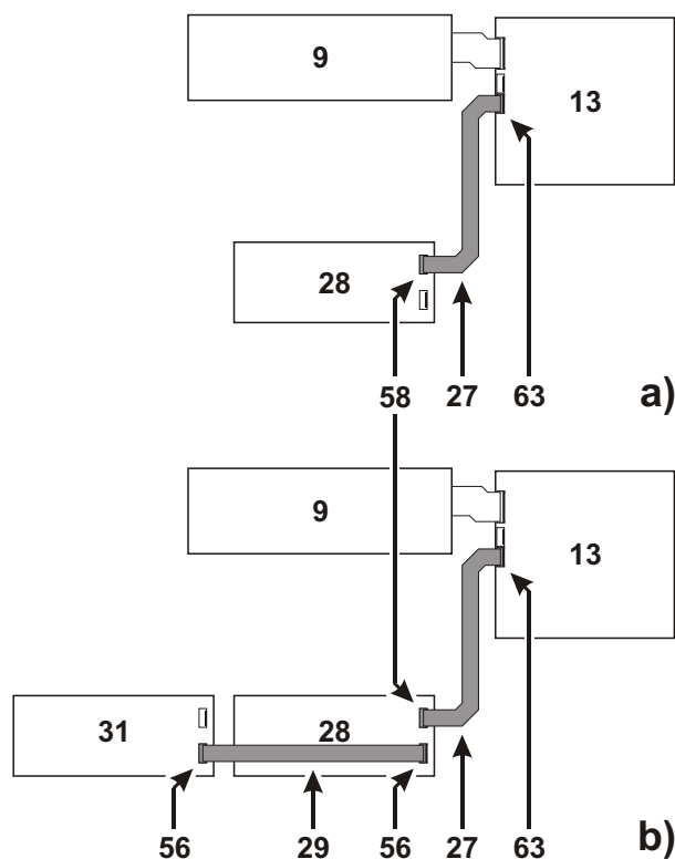
Figura 9 Conexión de UN Módulo de Extinción (a) o DOS Módulos de Extinción (b) a la Central J424: 9) Placa de Control Principal; 13) Placa Principal; 27) y 29) cable plano para conectar los Módulos de Extinción; 28) Módulo de Extinción n°. 1; 31) Módulo de Extinción n°. 2; 56) Conector para el Módulo de Extinción consecutivo 58) Terminal para conectar a la Placa Principal; 63) Conector para el Módulo de Extinción n°. 1.
