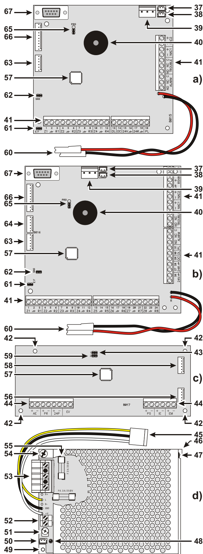
Figura 5 Identificación de Partes: a) Placa Principal (2 o 4 zonas); b) Placa Principal 8 zonas; c) Módulo Extinción; d) Fuente Alimentación conmutada de J408
