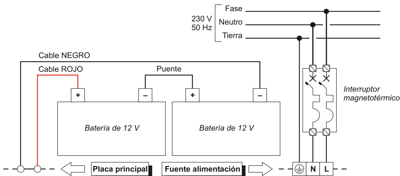
Figura 20 Conexión de la Alimentación
