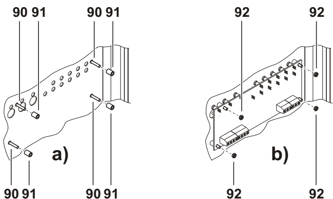
Figura 8 J424: Instalación del Módulo de Extinción
