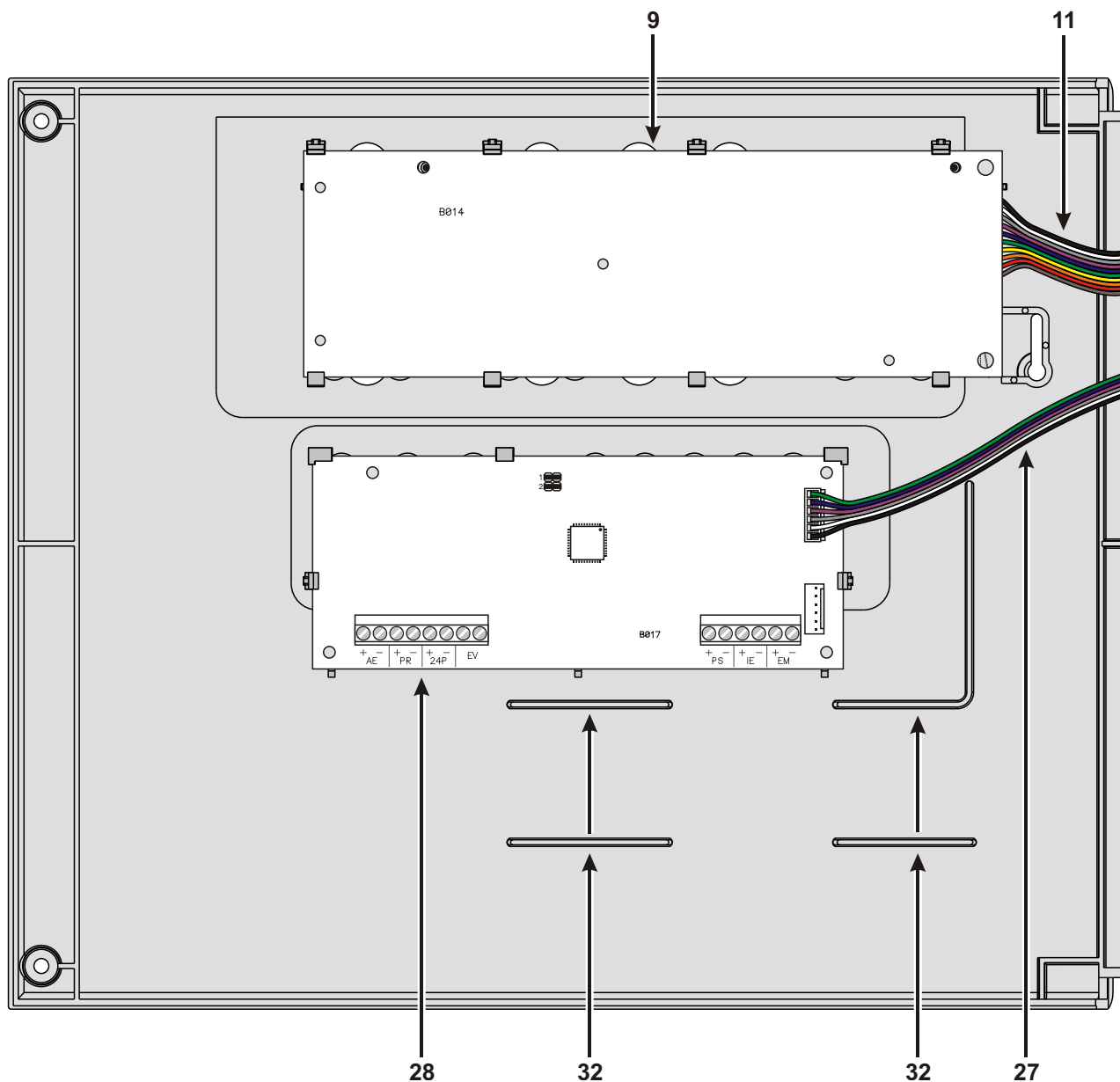
Figura 3 Configuración Máxima de la Central J408
