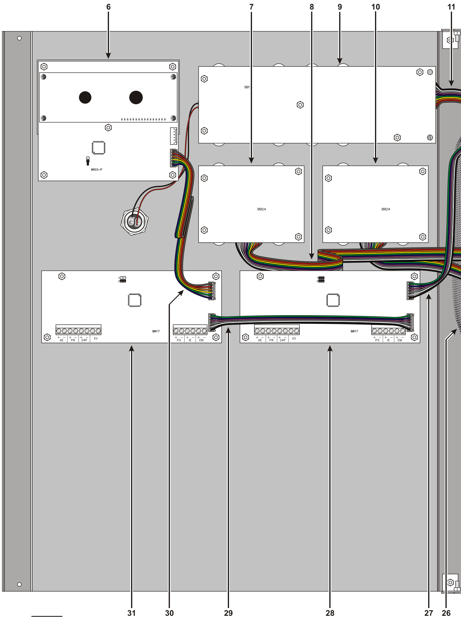
Figura 2 Máxima configuración de la Central J424
